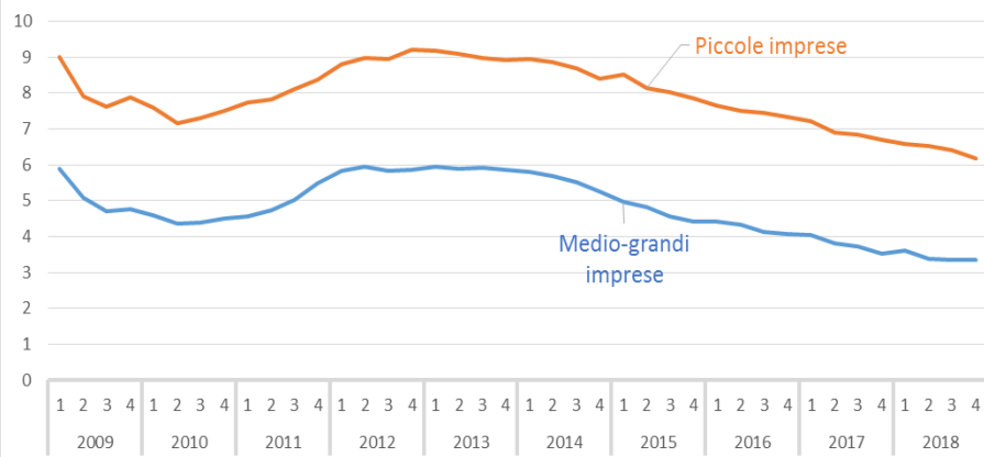
(B) Tassi di interesse a breve termine per dimensione delle imprese Lombardia, dati trimestrali 2009-2018
