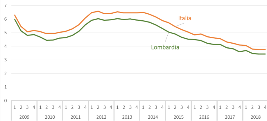
(A) Tassi di interesse a breve termine in Lombardia e in Italia Totale imprese, dati trimestrali 2009-2018
